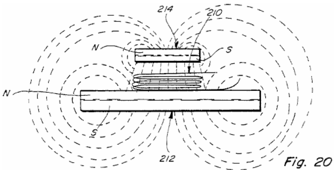
Fig.20 ist eine Seitenansicht ähnlich zu Fig.19 , zeigt jedoch eine zweite Permanentmagnet oberhalb des ersten Dauermagneten angeordnet und zeigt in gestrichelten Linien die magnetischen Felder der beiden Permanentmagnete, wenn kein elektrisches Potential über der Luftspule verbunden.
