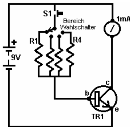
Transistor-Prüfer 3
