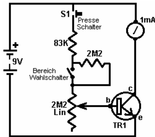
Transistor-Prüfer 2
