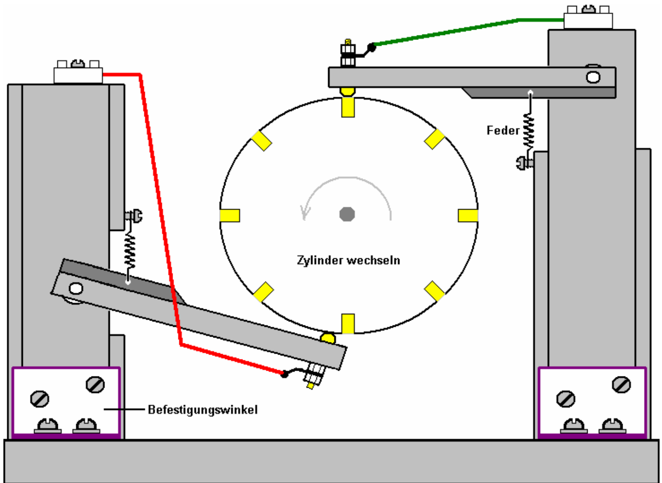
SEITENANSICHT
