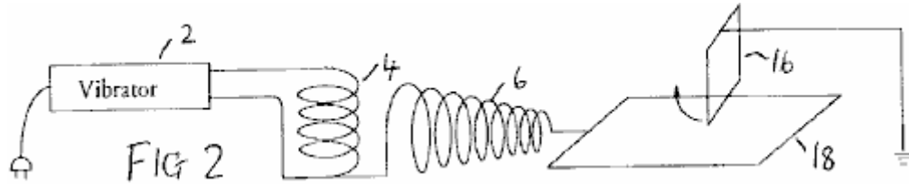
Fig.2 ist eine schematische Ansicht einer Tesla-Spule, um einen Goldelektrometer verbunden:
