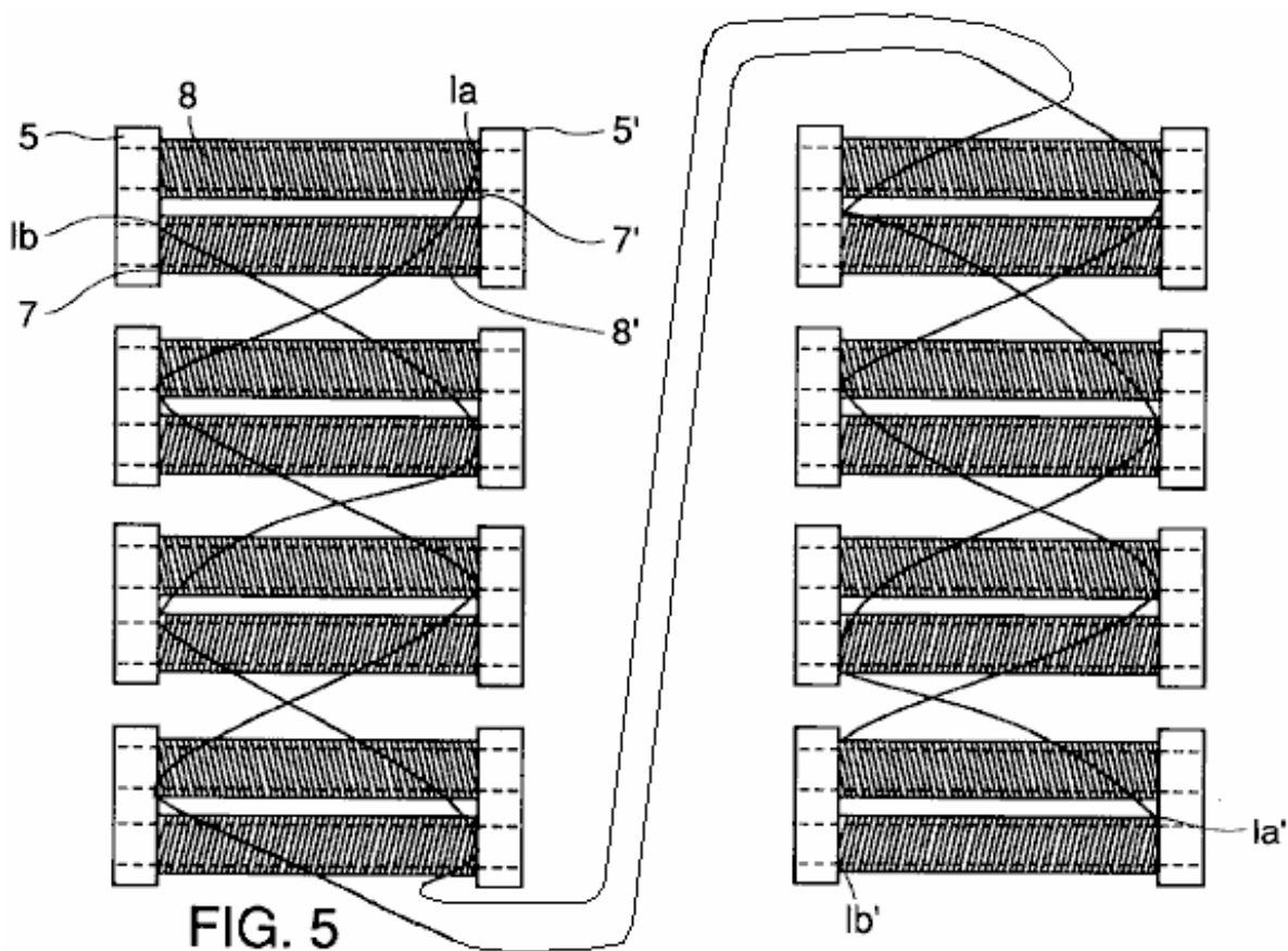
Fig.5 veranschaulicht eine Art der Verbindung magnetisch ansprechenden Spulen 7 und 7' um die magnetische Induktion tertiären Kerne 8 und 8' gewickelt mit acht Polen.
