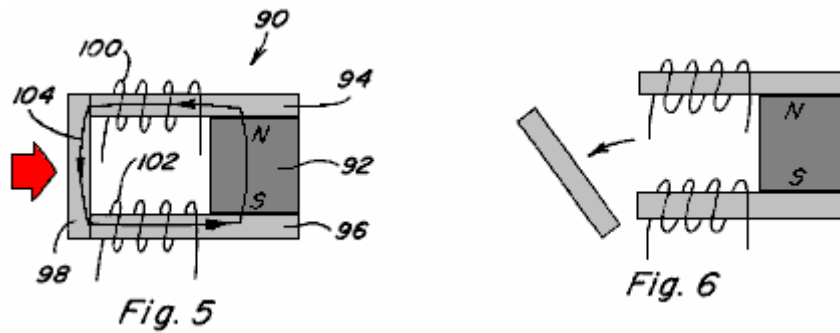
Fig.5 und Fig.6 sind Seitenansichten einer Permanentmagneteinrichtung einen Permanentmagneten mit Polschuhen gegen die Polflächen davon positioniert ist und einen beweglichen Anker;
