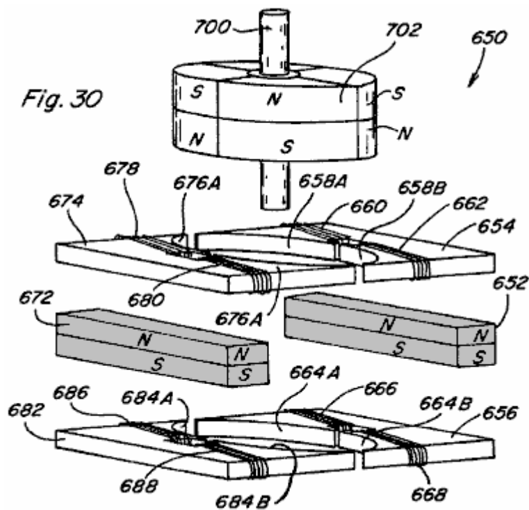
Fig.30 ist eine auseinandergezogene perspektivische Teilansicht einer anderen Ausführungsform einer Rotationsbewegungsrichtung;
