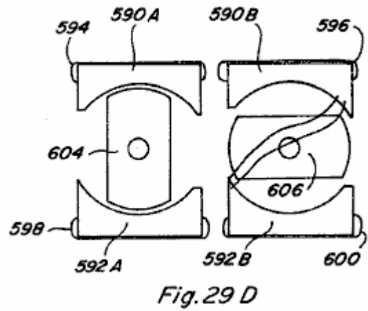
Fig.29A-Fig.29D Endansichten der Drehbewegungsrichtung von Fig.24 veranschaulicht eine Folge von seiner Drehbewegungen;
