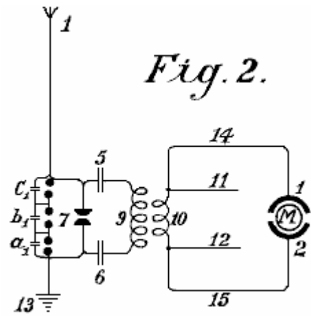
Fig.2 ist eine schematische Ansicht der einfachste Form.
