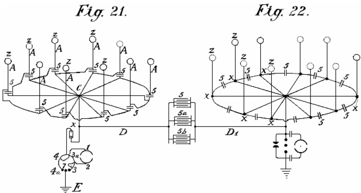
Fig.21 zeigt schematisch eine Anordnung zum Sammeln von großen Energiemengen,.
