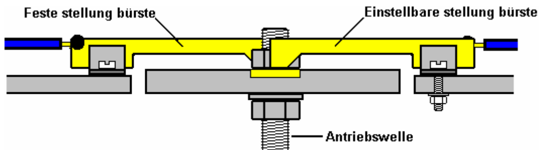
STEUERUNG - SEITENANSICHT
