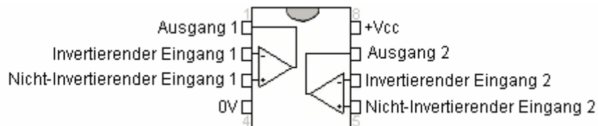
LM358
