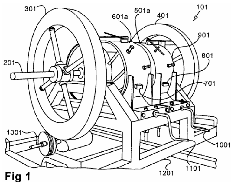
Fig.1 ist eine perspektivische Ansicht der Haube-Verkörperungen des magnetischen Motors mit Schwungräder befestigt.
