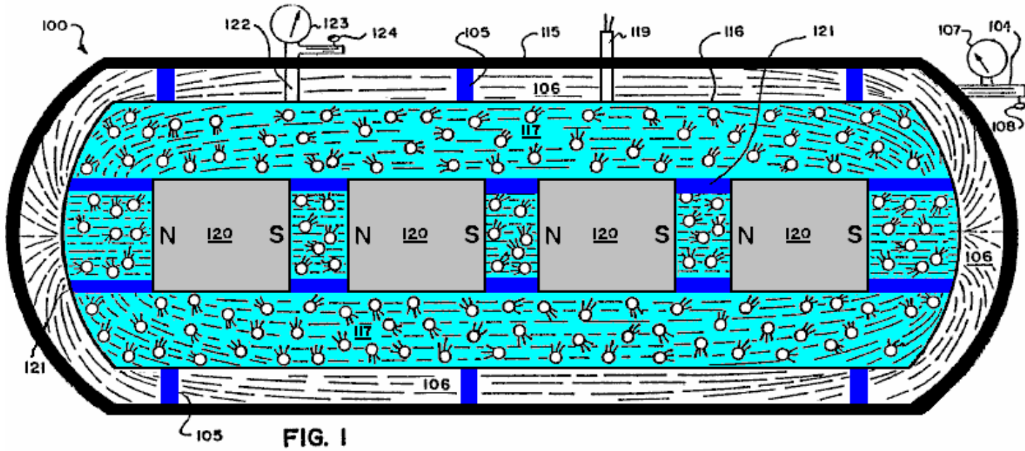
Fig.1 ist eine schematische Seitenansicht in allgemeiner, Darstellungsform einer ersten Ausführungsform eines elektrischen Generators auf der Grundlage der Grundsätze und Leitlinien der vorliegenden Erfindung.
