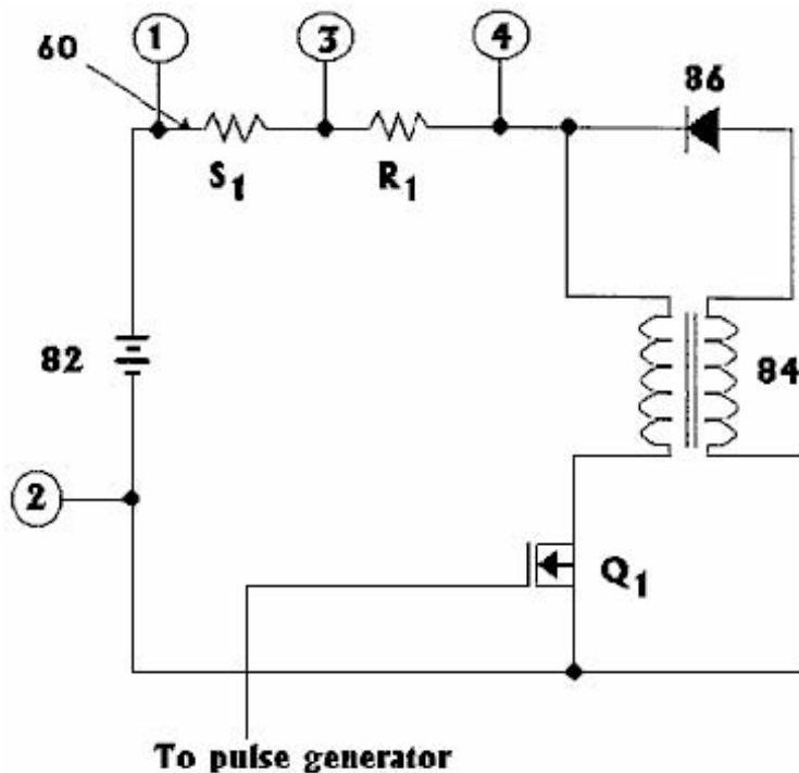
Fig.4 zeigt die Testschaltung in Beispiel 2 unten beschrieben.
