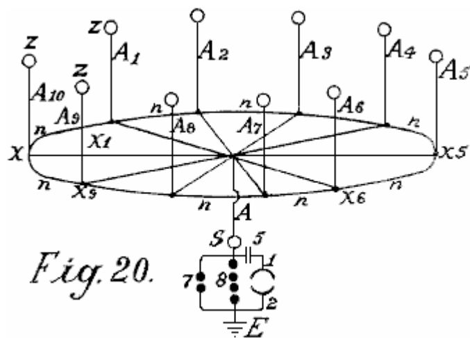
Fig.20 zeigt eine einfache Form, in der die Antenne Netzwerk ist mit speziellen Kollektoren kombiniert
