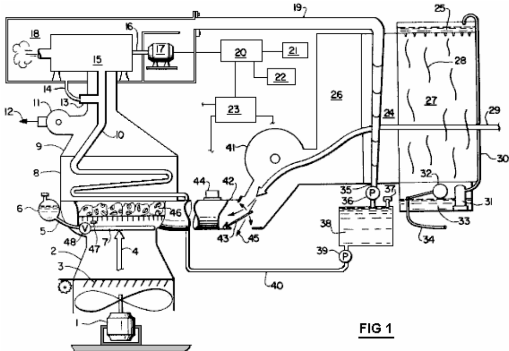
Fig.1 ist eine teilweise geschnittene schematische Ansicht des Systems:
