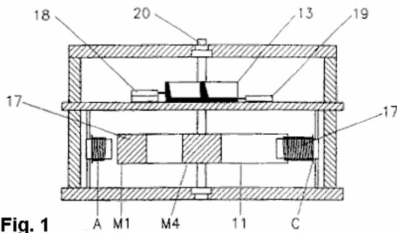
Fig.1 zeigt eine Querschnittsvorderansicht einer Drehvorrichtung als Steuer daher in Übereinstimmung mit einer ersten Ausführungsform der Erfindung;
