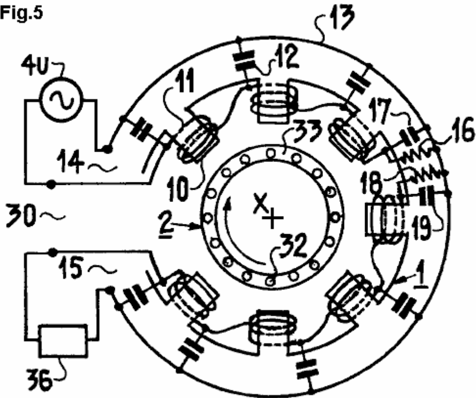
Fig.5, eine schematische Darstellung einer Variante der Maschine nach der Erfindung mit einem Stator gemäß dem Design der Fig.2;
