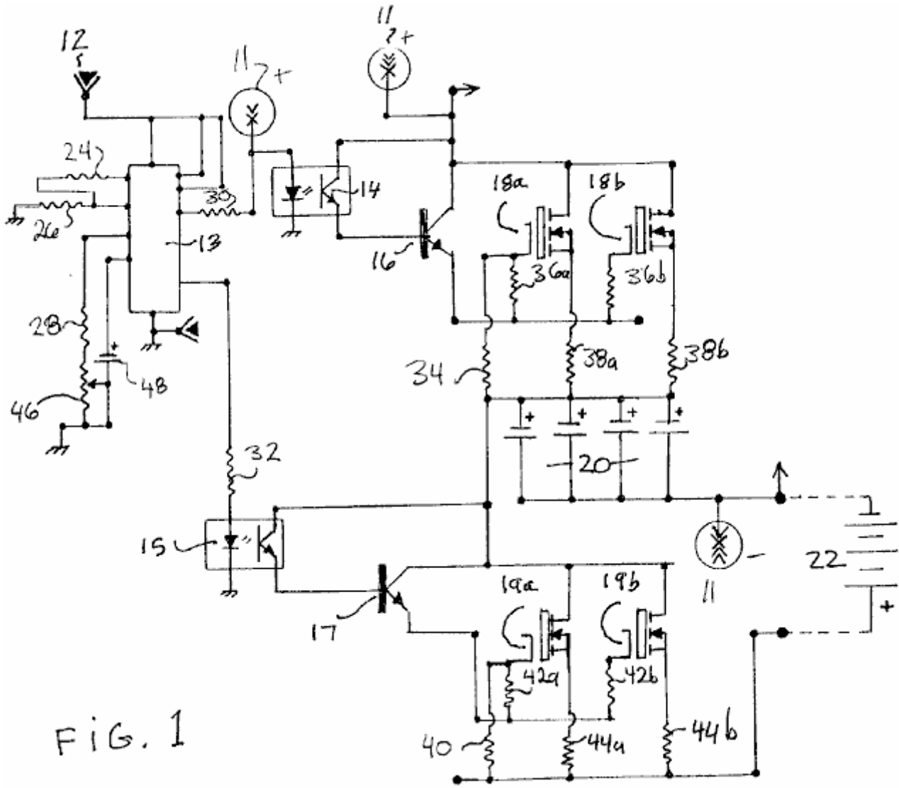
Fig.1 ist eine schematische Darstellung eines Festkörperimpuls-ladegerät gemäß einem Ausführungsbeispiel der Erfindung.
