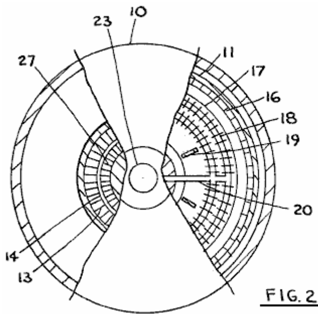
Fig.2 ist eine Endansicht der Einheit im gezeigten Fig.1.
