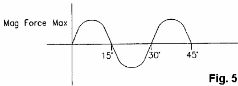
Fig.5 zeigt eine graphische Darstellung der Kraft über der Winkelposition des Permanentmagneten M1 des in Fig.4A gezeigten Systems;
