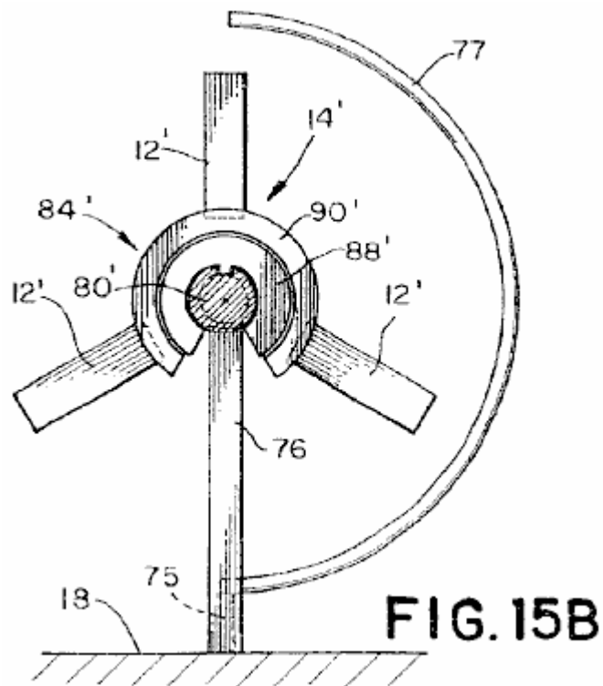
Fig.15B ist eine Stirnansicht der vierzehnten Ausführungsform gezeigt in Fig.15A;
