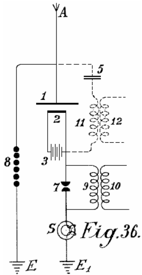
Fig.36 zeigt eine glühende Sammler mit Nernstlampe
