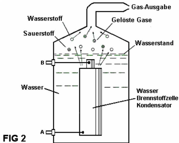
Fig.2 zeigt eine Perspektive auf ein "Wasser-Kondensator" Element in der Brennstoffzelle-Schaltung.
