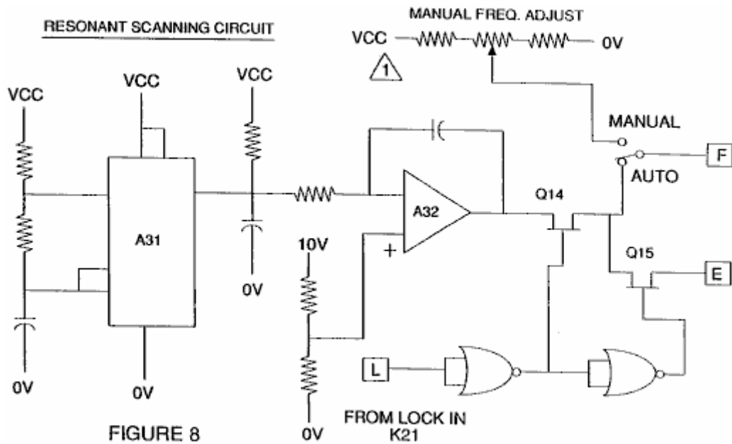
Fig.8 eine Resonanz Abtastschaltung
