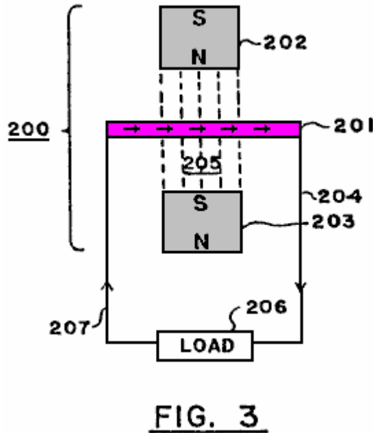
Fig.3 ist eine schematische Ansicht in generalidarstellungsform einer zweiten Ausführungsform eines elektrischen Generators, basierend auf den Prinzipien und Richtlinien der vorliegenden Erfindung.
